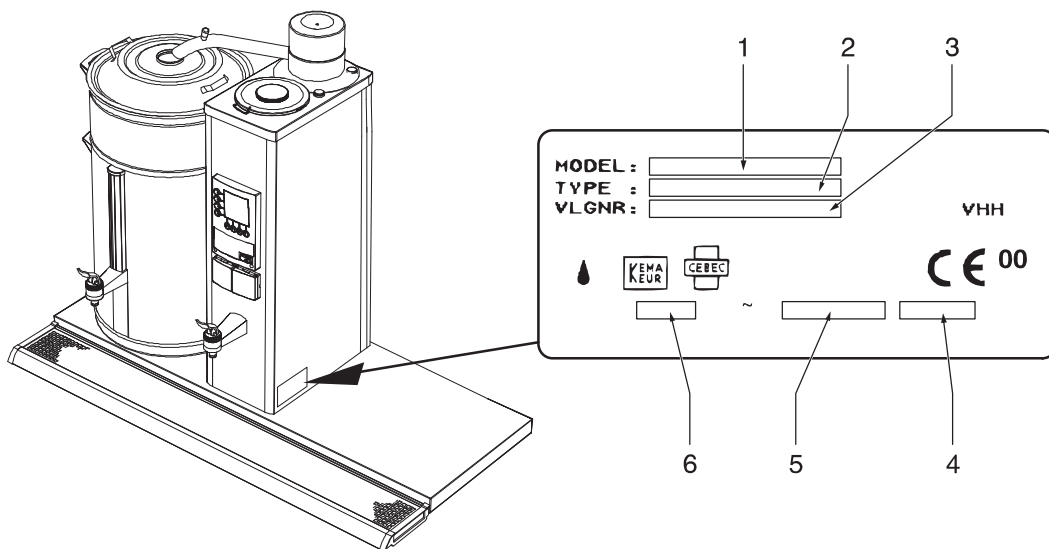
Fig. 1 Märkbricka
