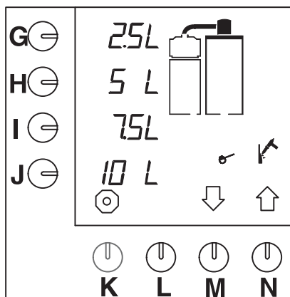
Fig. 4 Display med avkalkningssignal kaffebryggarsystem
