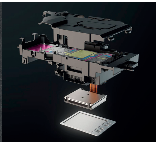
1 680 enskilda bläckkammare Δ
